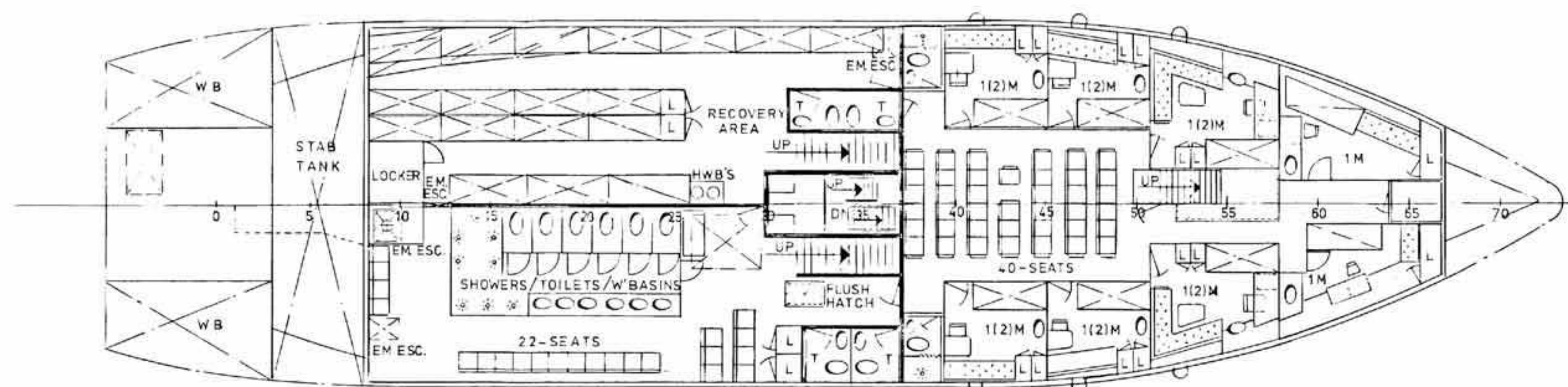
TWEEN DECK
